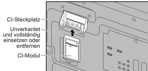
Rückseite des Fernsehers
