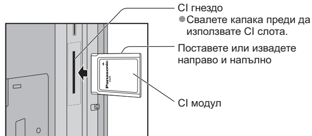
Страничен панел на телевизора
