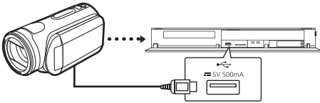
USB-Anschlusskabel (Sonderzubehör)
